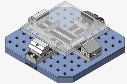
Beispiel 3 auf Rasterplatte 500x500x40 Example 3 on grid plate 500x500x40
