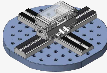
Beispiel 2 auf Rasterplatte rund Ø500 x 40 Example 2 on grid plate round Ø500 x 40
