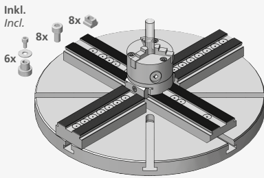
Beispiel 1 auf 5-Achs Maschinentisch Example 1 on 5-axis machine table
